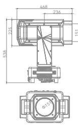
顶视图
